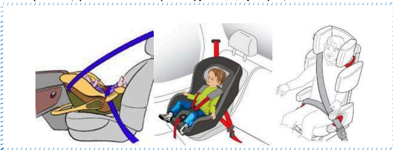
Рисунок 4. Крепление штатными ремнями безопасности
